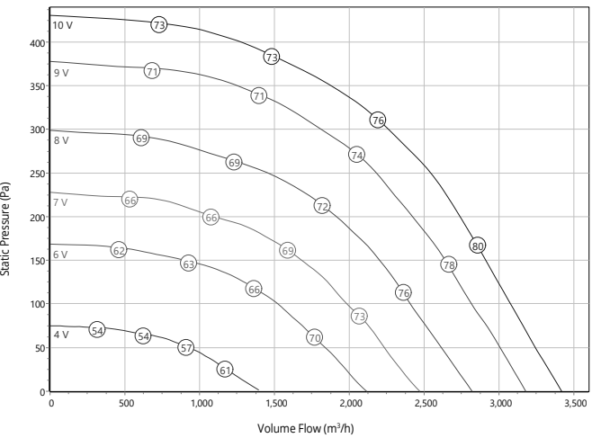
KATANA EC 400-1 - RE400003
