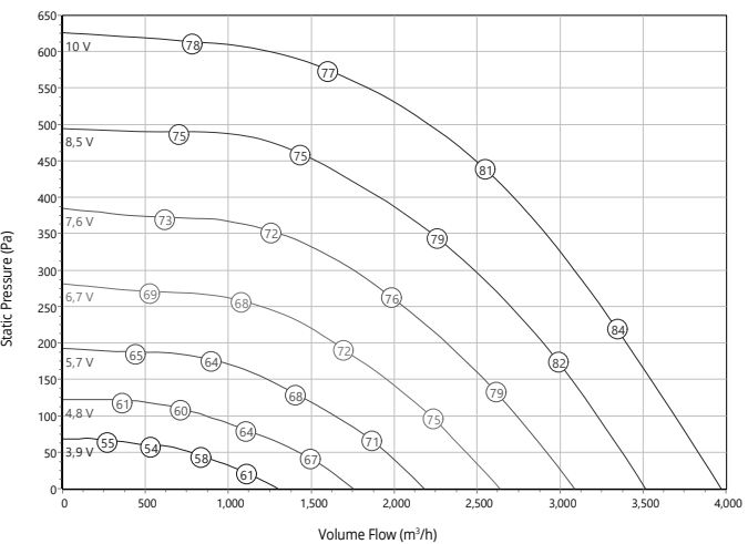
Katana EC 400-3 - RE400005
