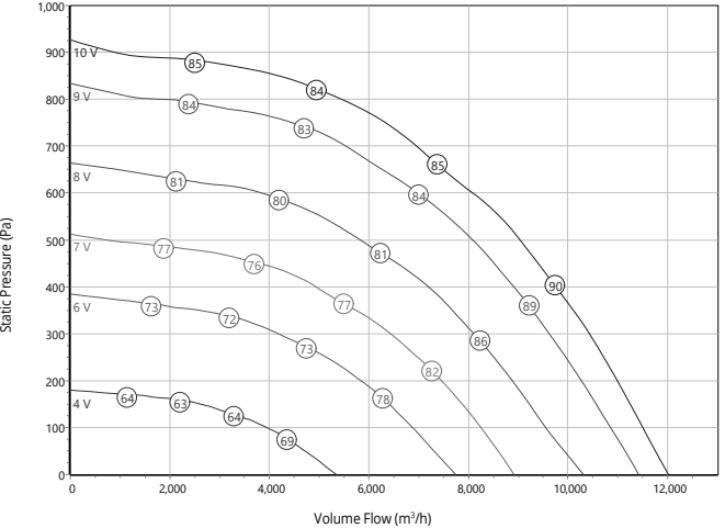
KATANA EC 560-3 - RE560004
