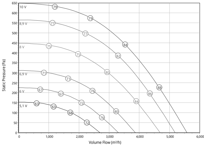
KATANA EC 355-3 - RE355007
