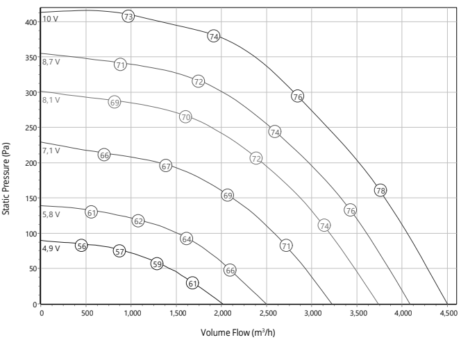
ESTOC TARGE EC 67-450-1 - GF674506
